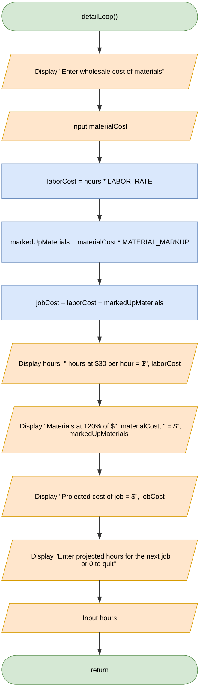
detailLoop() Module
