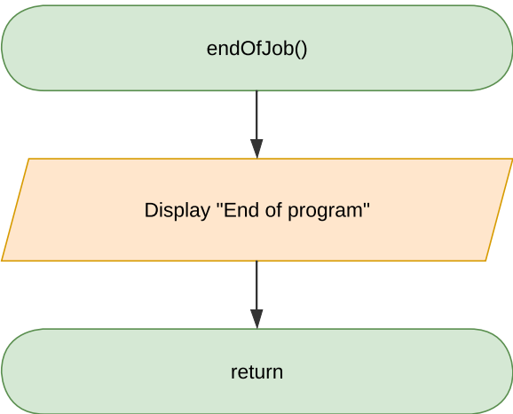
endOfJob() Module
